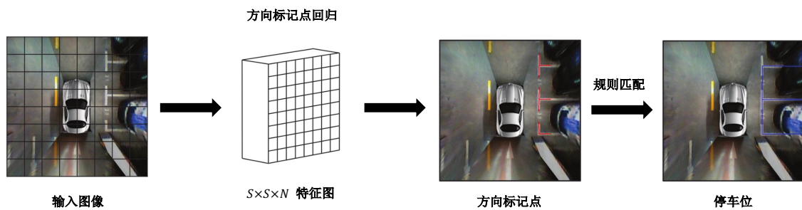
图 1-2 DMPR-PS [19] 算法流程图
