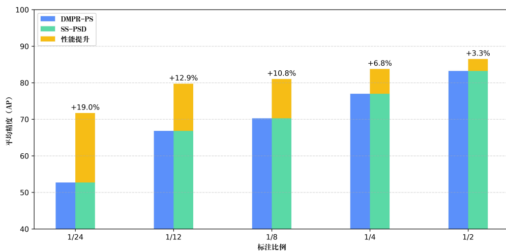
图 3-8 CRPS-D 数据集上 SS-PSD 与 DMPR-PS [19] 的性能对比
