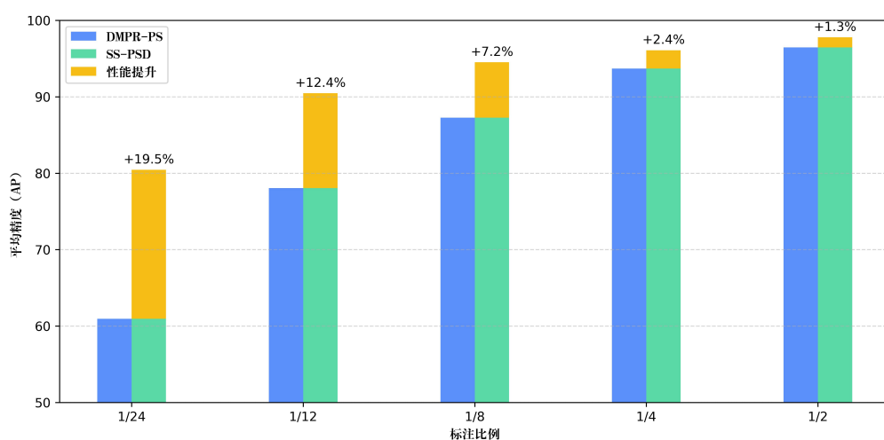
图 3-7 ps2.0 数据集上 SS-PSD 与 DMPR-PS [19] 的性能对比
