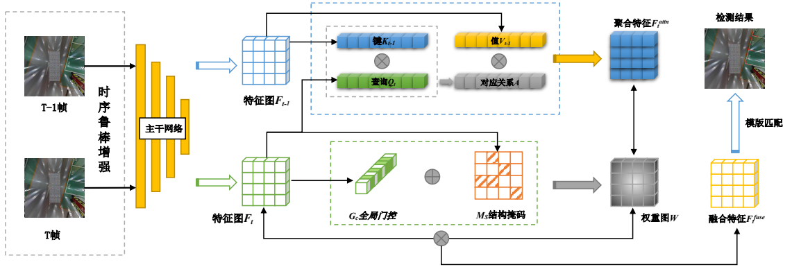
图 5.1 面向多帧时序信息融合的停车位检测方法示意图
