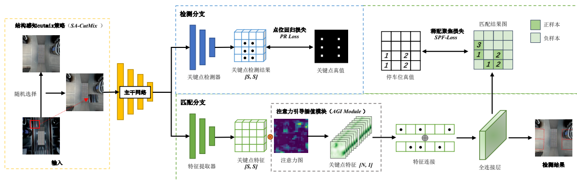
图 4.1 面向结构感知的停车位关键点检测与匹配方法示意图
