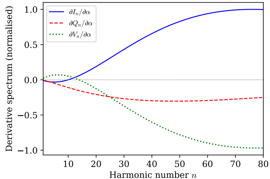
(d) Pitch-angle derivative ( \alpha_0 = \pi/4 )
