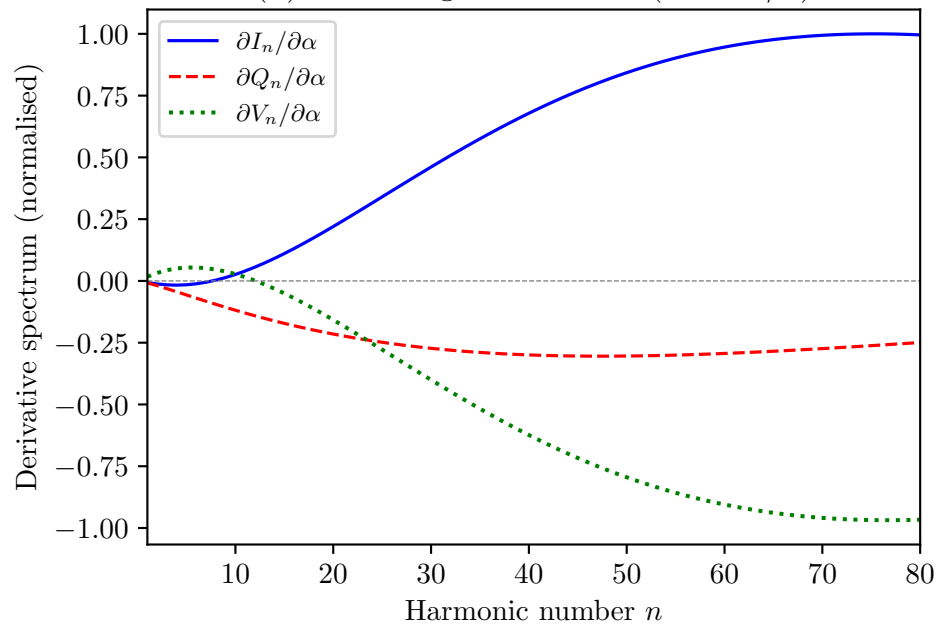
(d) Pitch angle derivative ( \alpha_0 = \pi/4 )
