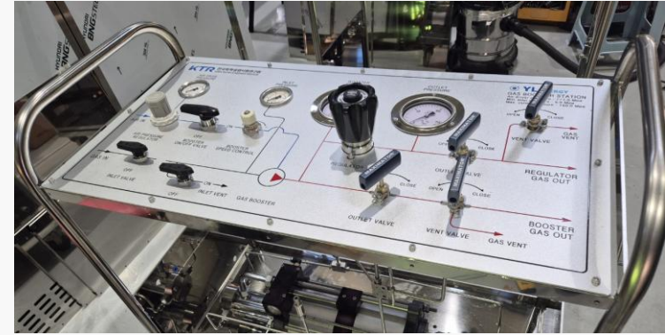
<100MPa급 2단 수소가압시스템(KTR)>
