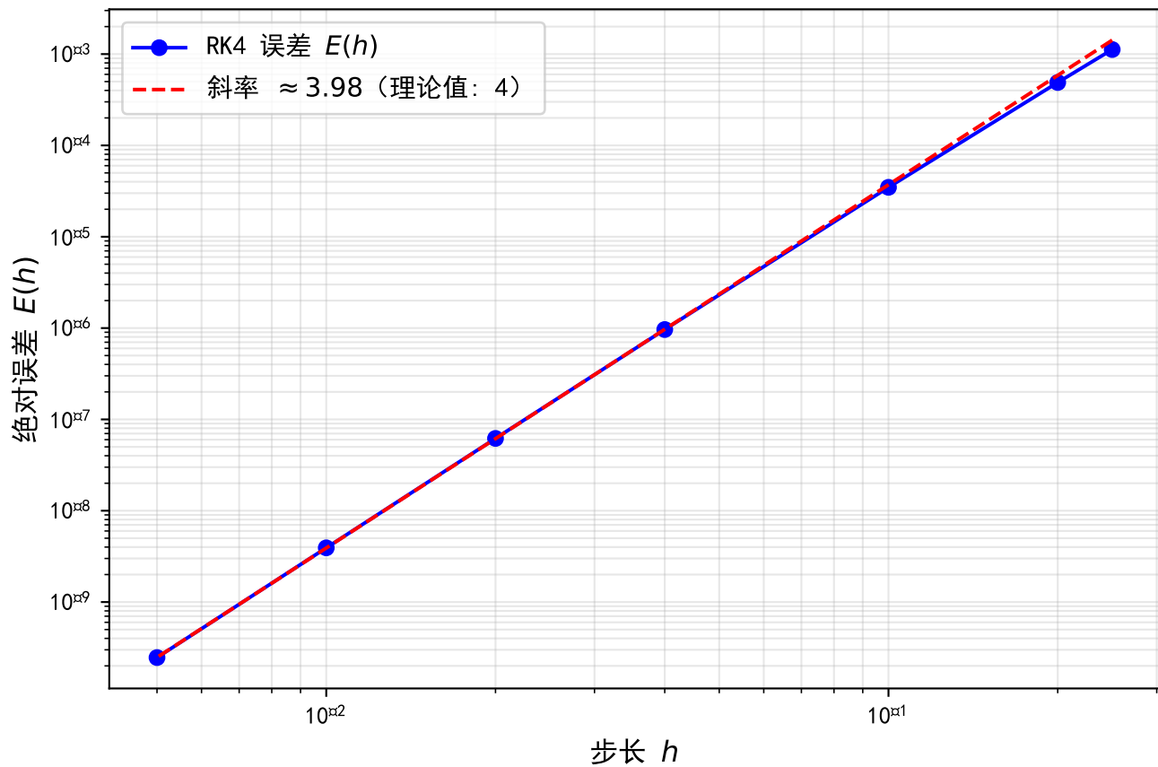
RK4 方法收敛阶分析
