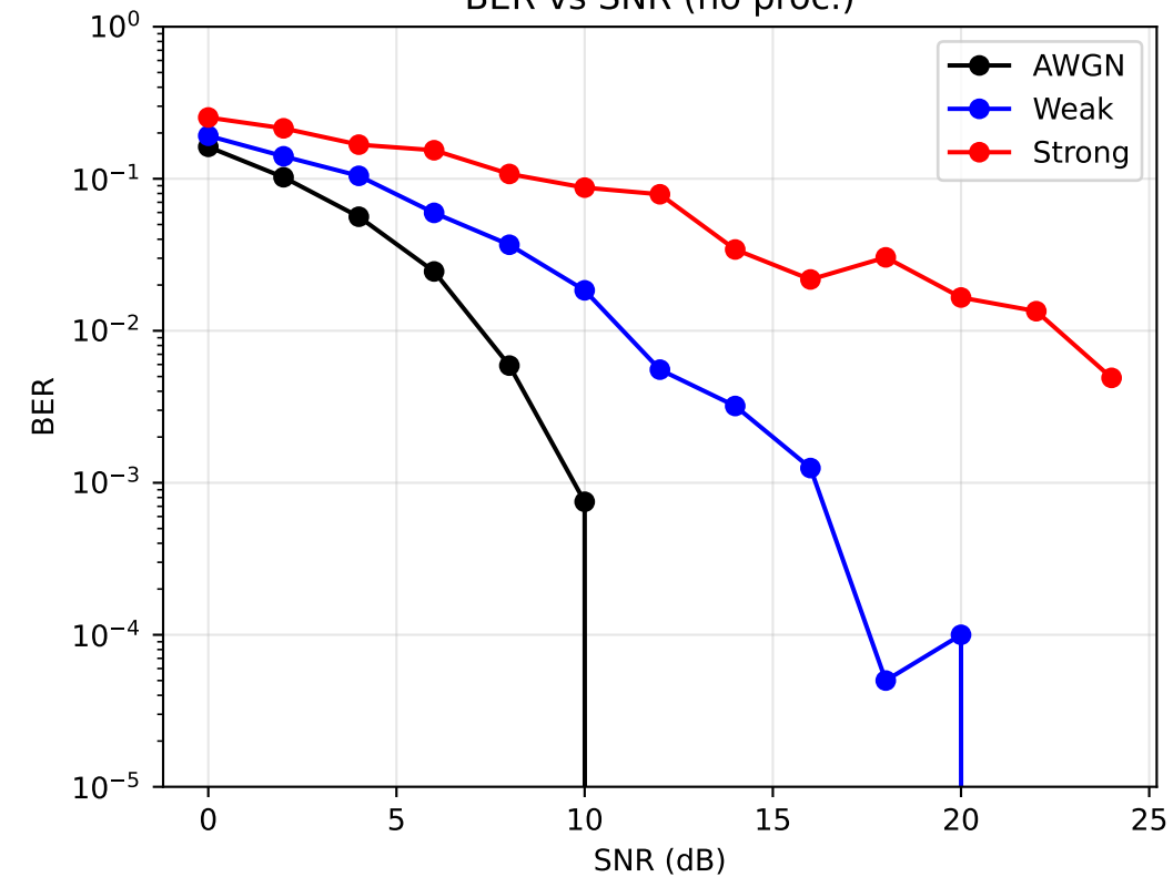
BER vs SNR (no proc.)
