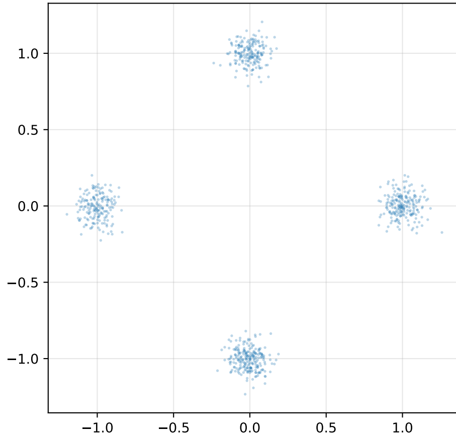
After VV (BER=0.0000)
