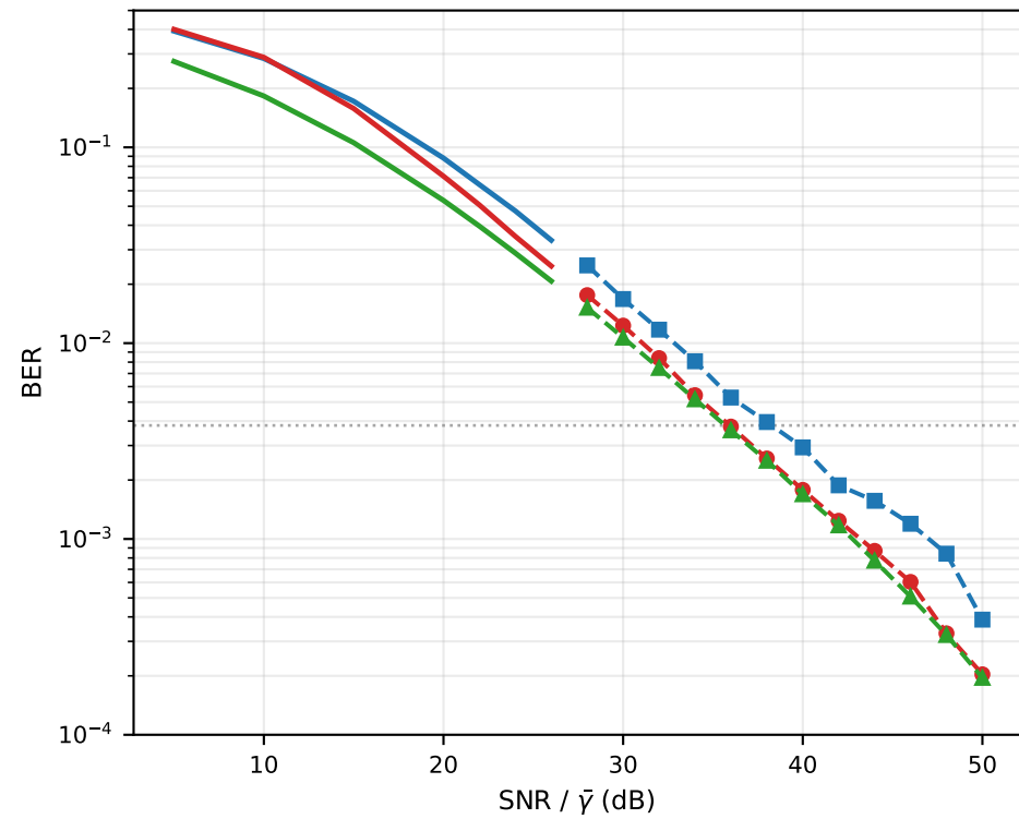
(d) Strong turb. ( \alpha=1.5, \beta=0.8 )
