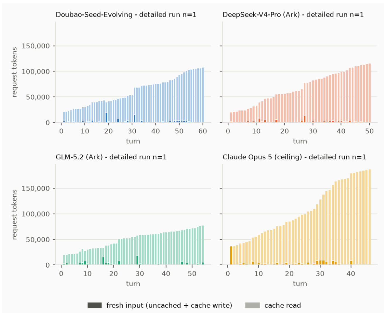
图 2：上下文增长（详细版，逐轮）
