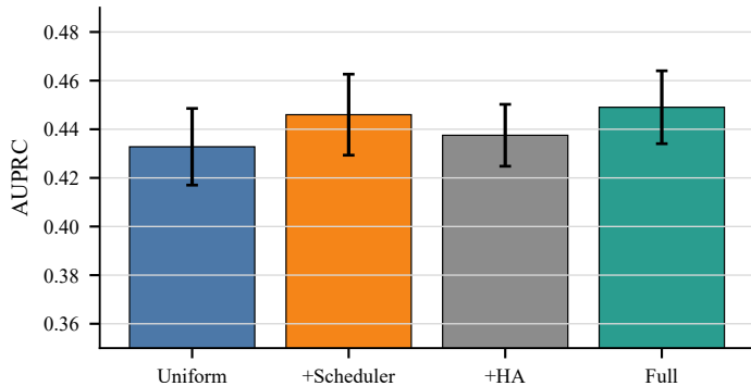
Dirichlet \alpha = 0.5
