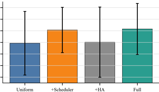
Dirichlet \alpha = 0.1
