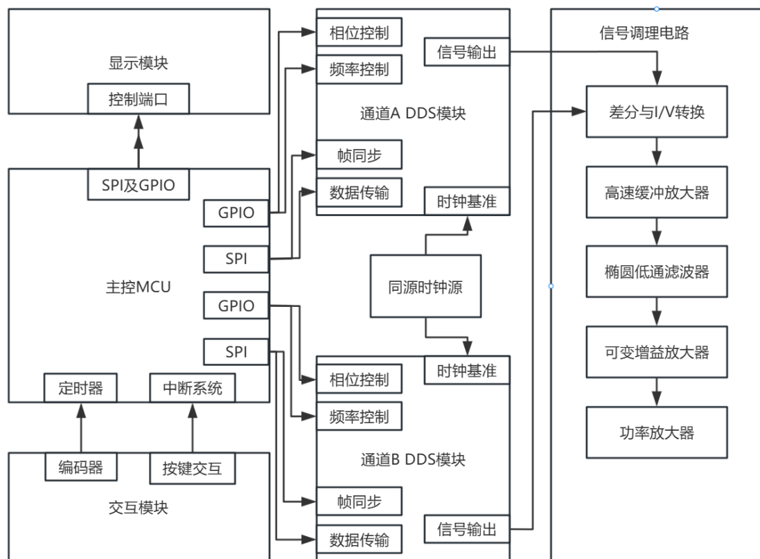
图 2- 1 系统设计方框图
