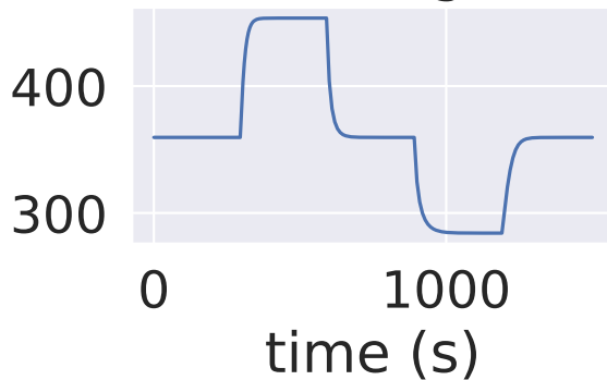
sCO 2 out (kg/m 3 )
