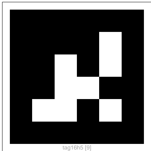
tag16h5 [9]
