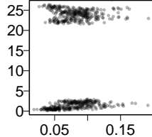
UMAP-U, 10
