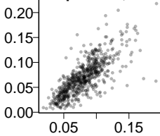
UMAP-S, 5
