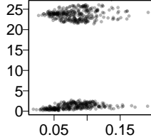
UMAP-U, 20
