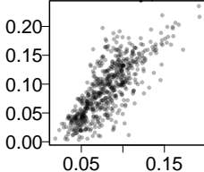
Isomap, 5
