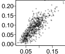
Isomap, 7
