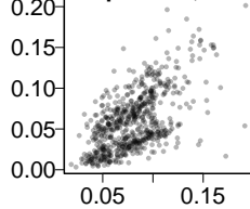
UMAP-S, 20
