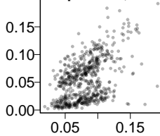
UMAP-S, 30
