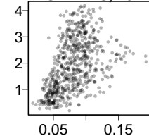
t-SNE, 10
