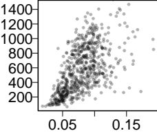
Isomap, 7
