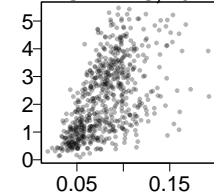
t-SNE, 7
