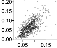
UMAP-S, 10
