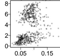
t-SNE, 5
