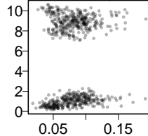
UMAP-U, 30
