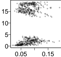
UMAP-U, 5
