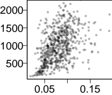
Isomap, 5
