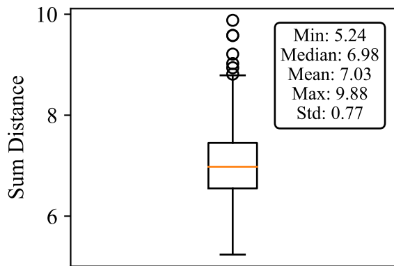
(d) GPT3.5
