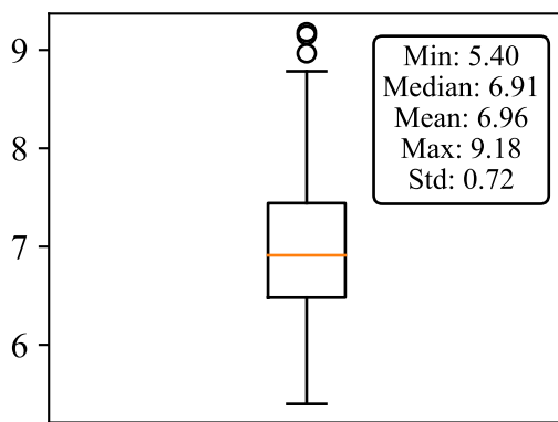
(e) GPT4
