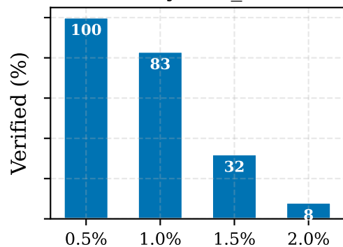
Layer fc_6
