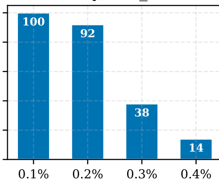
Layer fc_5
