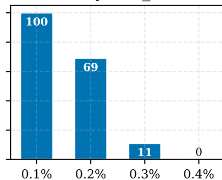
Layer fc_4
