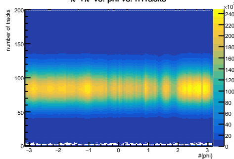
\pi^+\pi^- vs. \phi vs. nTracks
