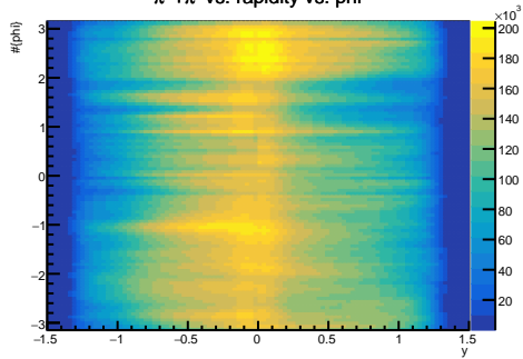
\pi^+\pi^- vs. rapidity vs. \phi
