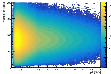
\pi^+\pi^- vs. p_T vs. nTracks
