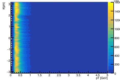
\pi^+\pi^- vs. p_T vs. \phi
