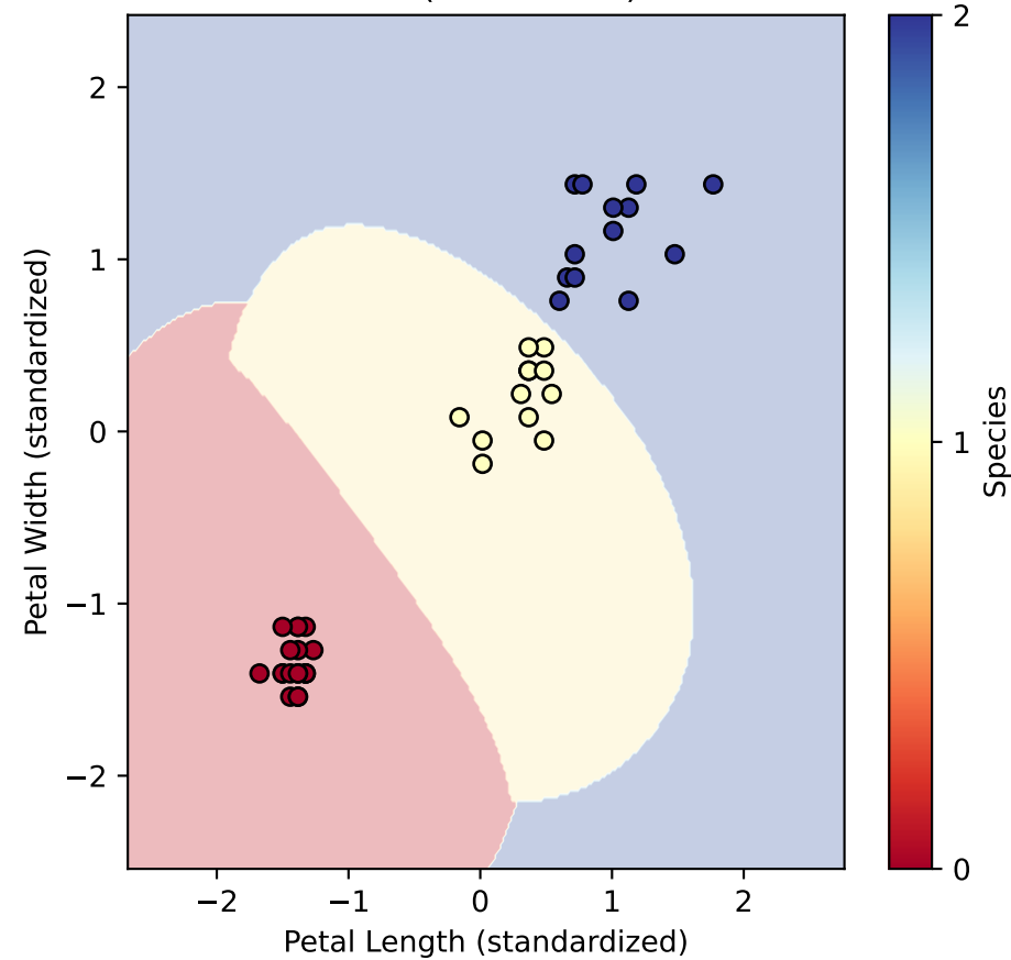
SVM (RBF Kernel)
