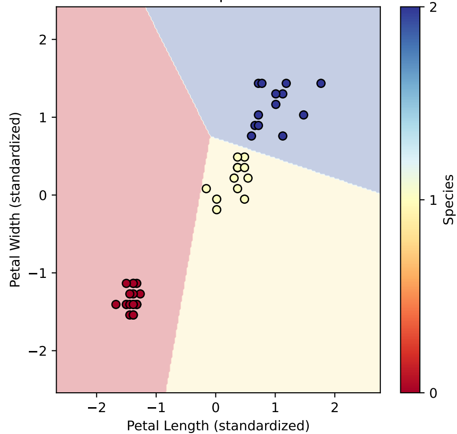
Perceptron
