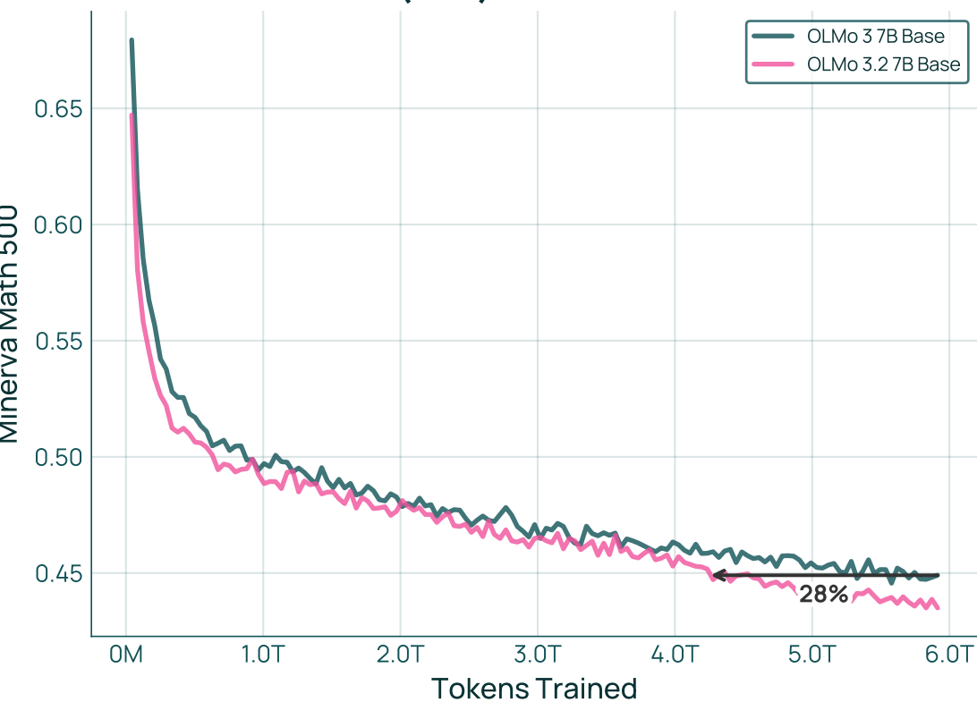
Minerva Math 500 (BPB)
