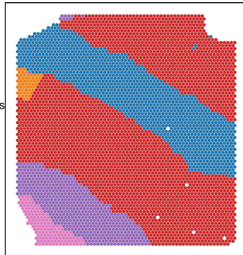
K = 5
