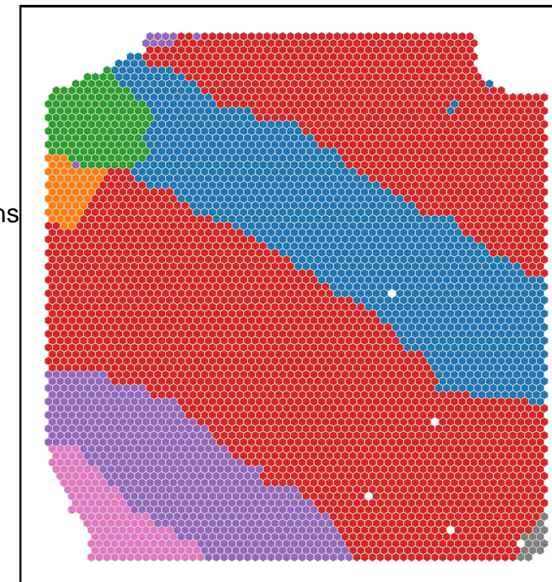
K = 7
