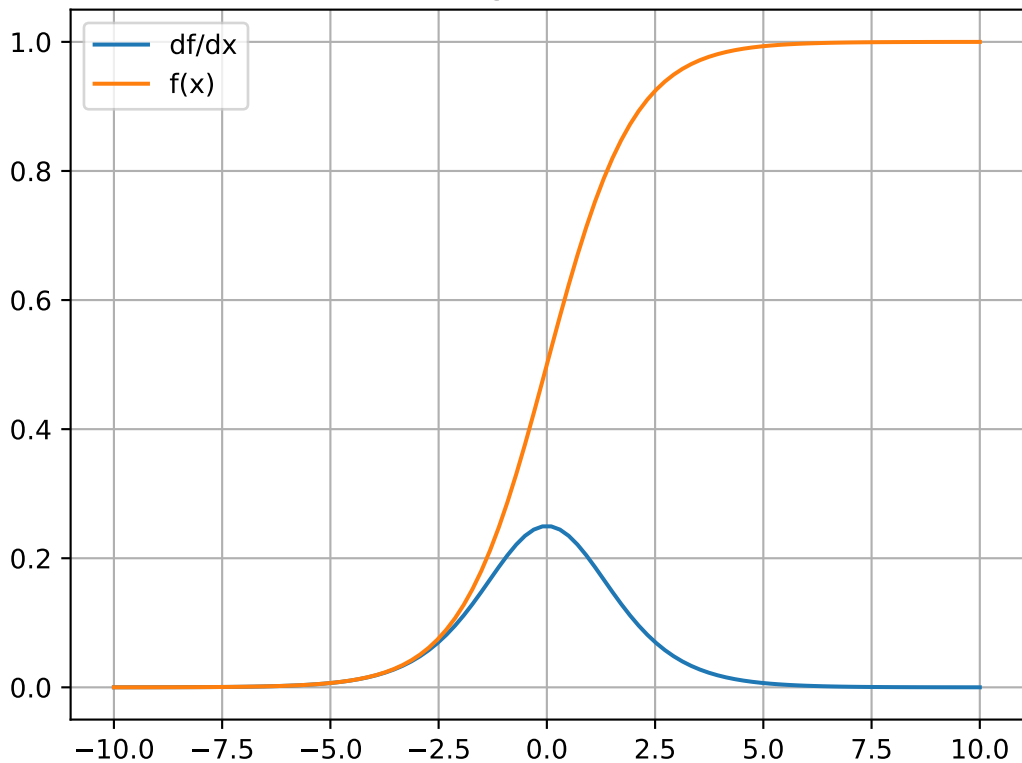
sigmoid(x)
