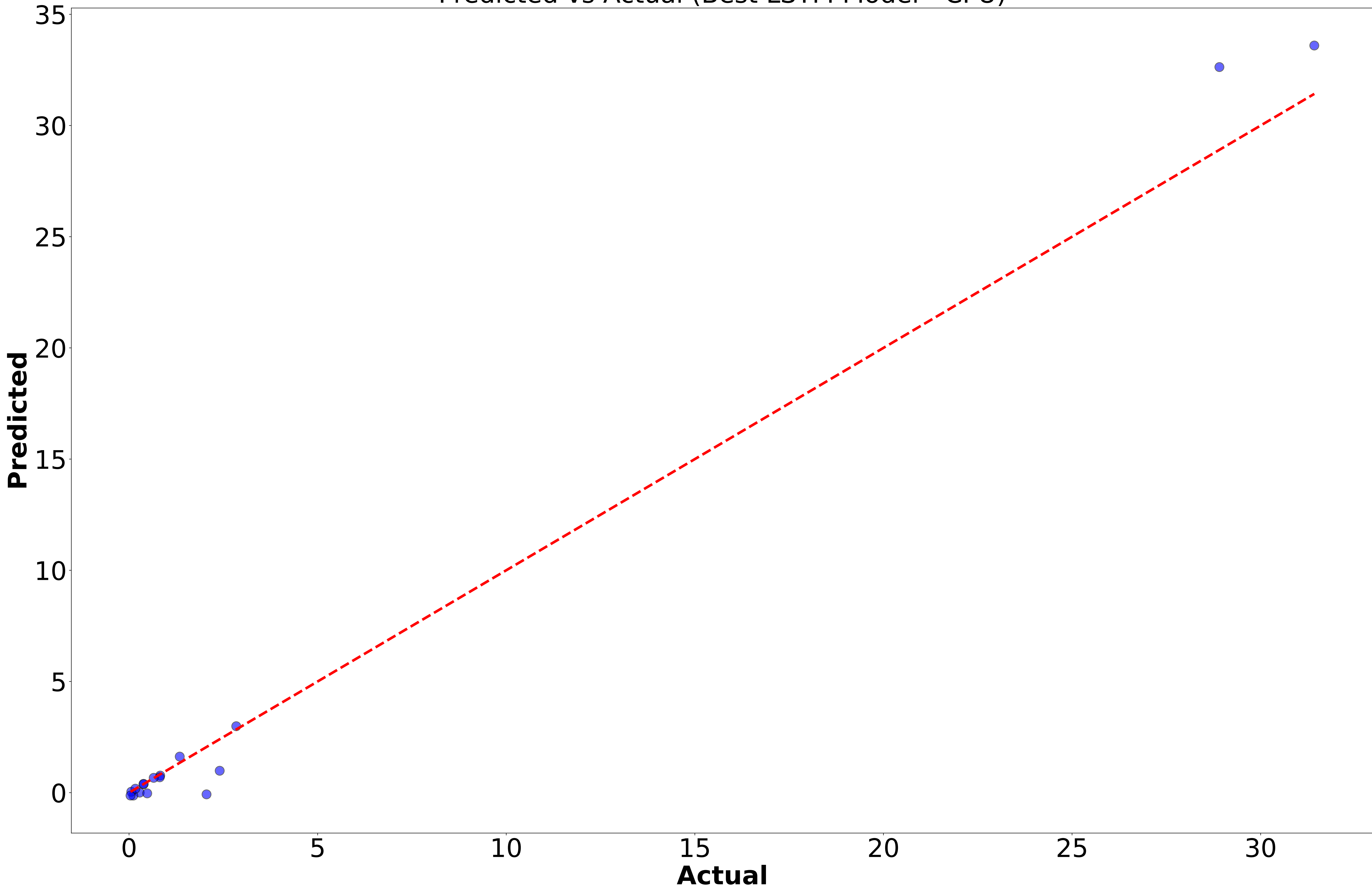
Predicted vs Actual (Best LSTM Model - CPU)
