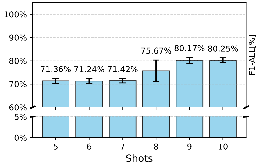
Edge-IIoT
