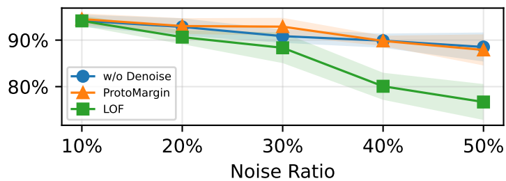
F1-ALL
