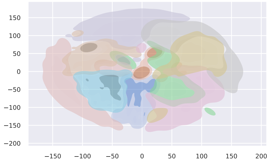
NN-Denoise
