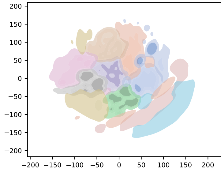
NN-Denoise
