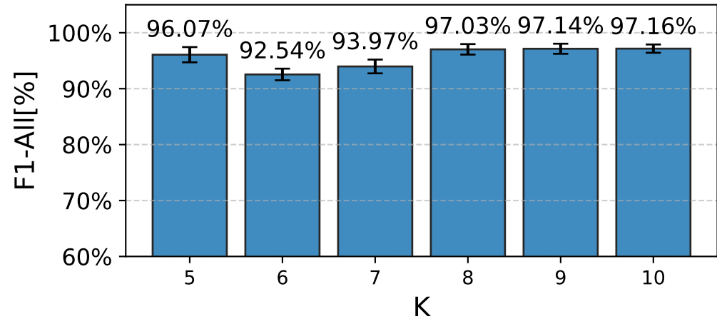
CSE-CIC-IDS2018
