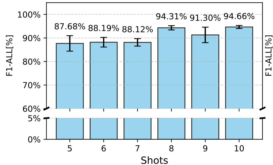
CSE-CIC-IDS2018
