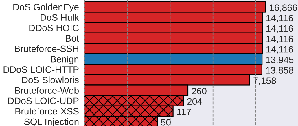
CSE-CIC-IDS2018
