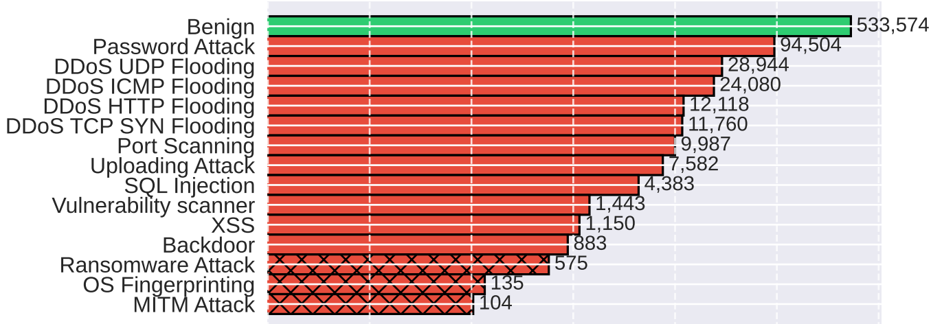
Edge-IIoT
