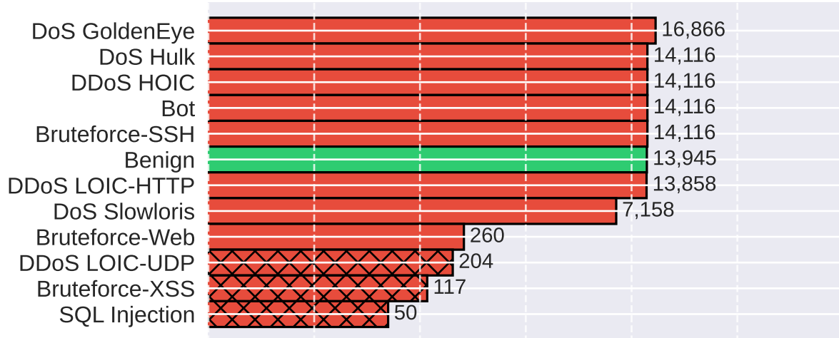
CSE-CIC-IDS2018
