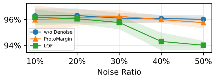
F1-Old
