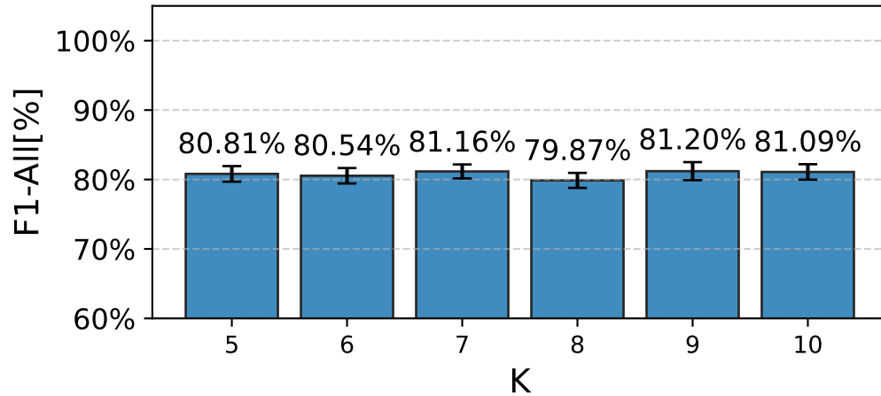
Edge-IIoT
