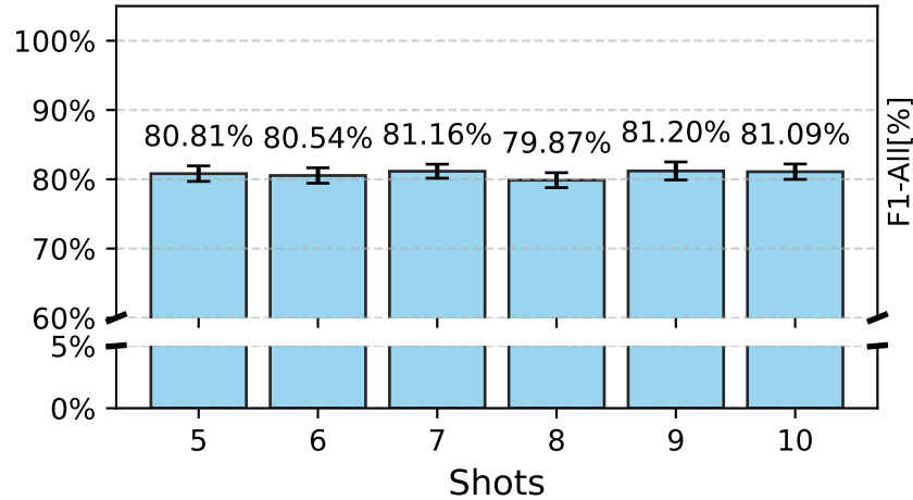
Edge-IIoT
