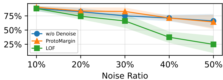
F1-New
