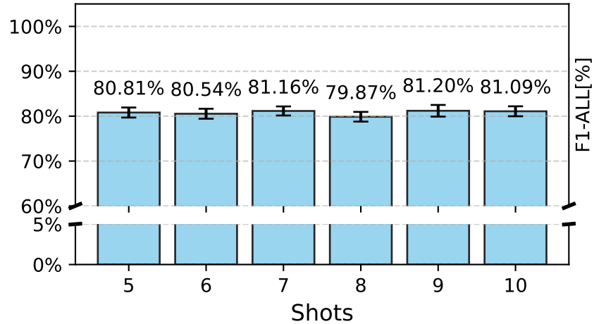
Edge-IIoT
