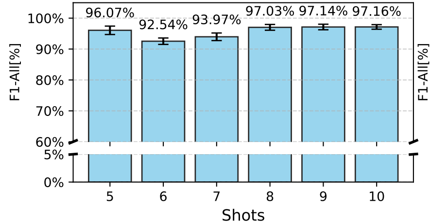
CSE-CIC-IDS2018
