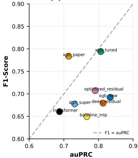
(b) F1 vs auPRC
