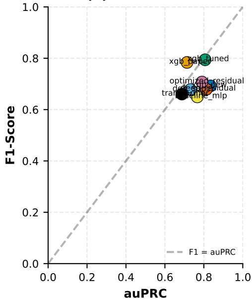
(b) F1 vs auPRC
