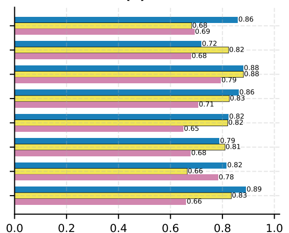
(e) F1
