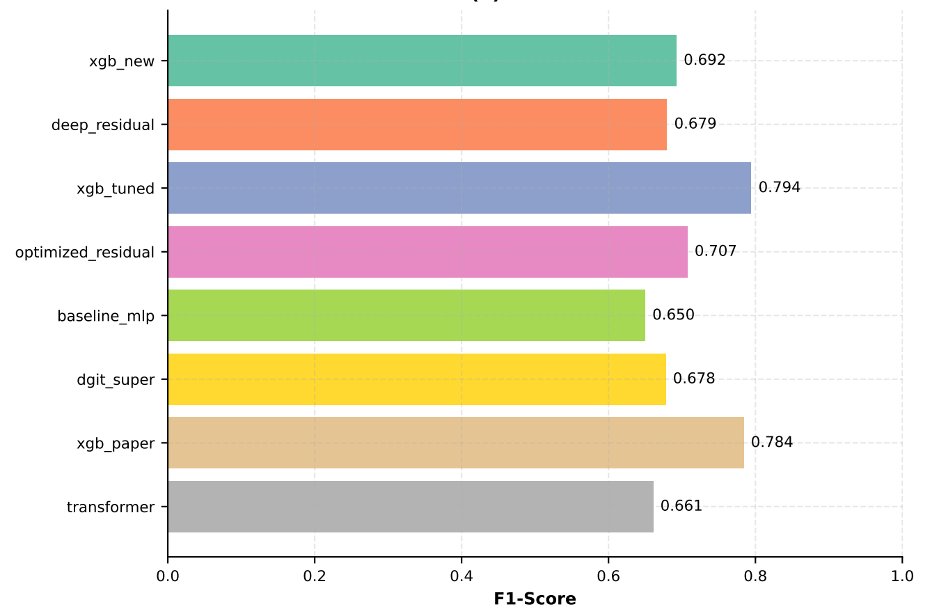
(d) F1-Score
