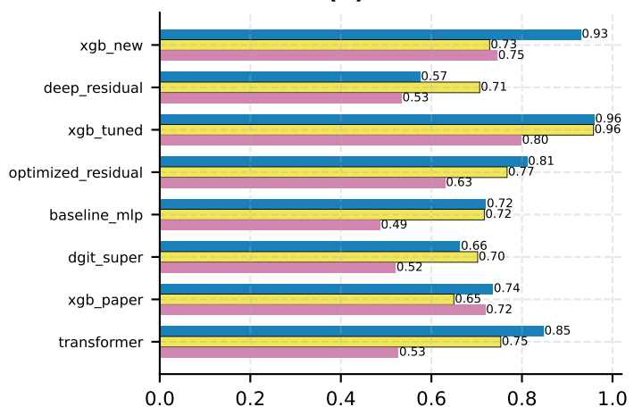
(d) Recall
