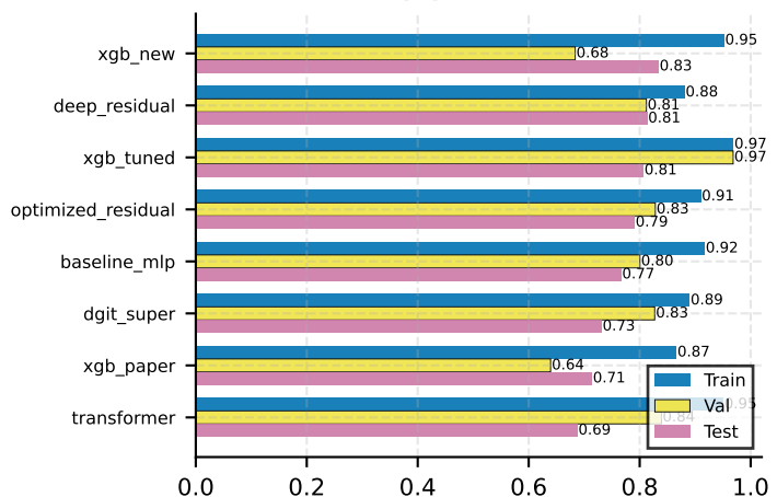
(a) auPRC
