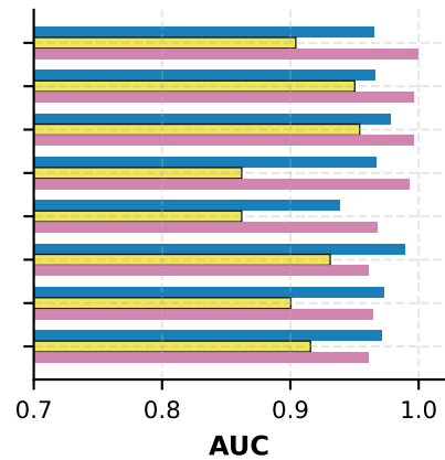
(f) AUC
