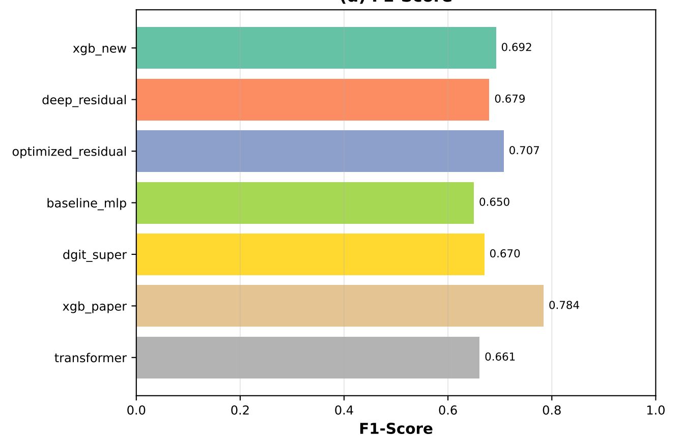
(d) F1-Score
