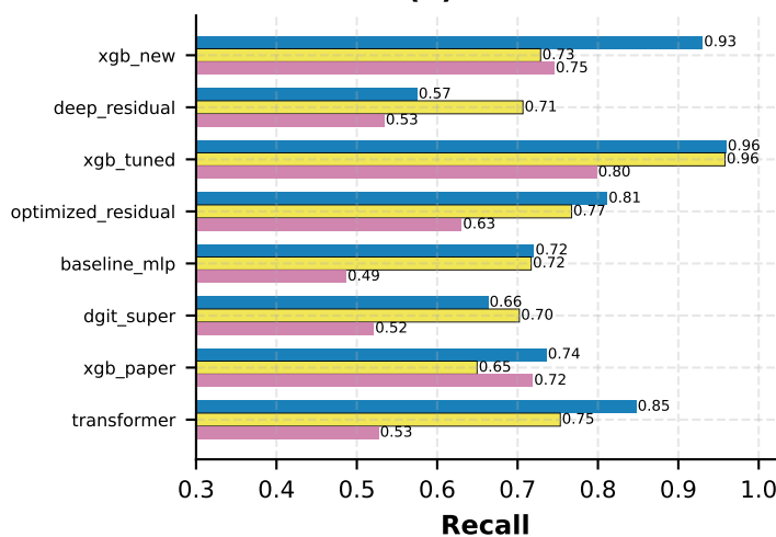
(d) Recall
