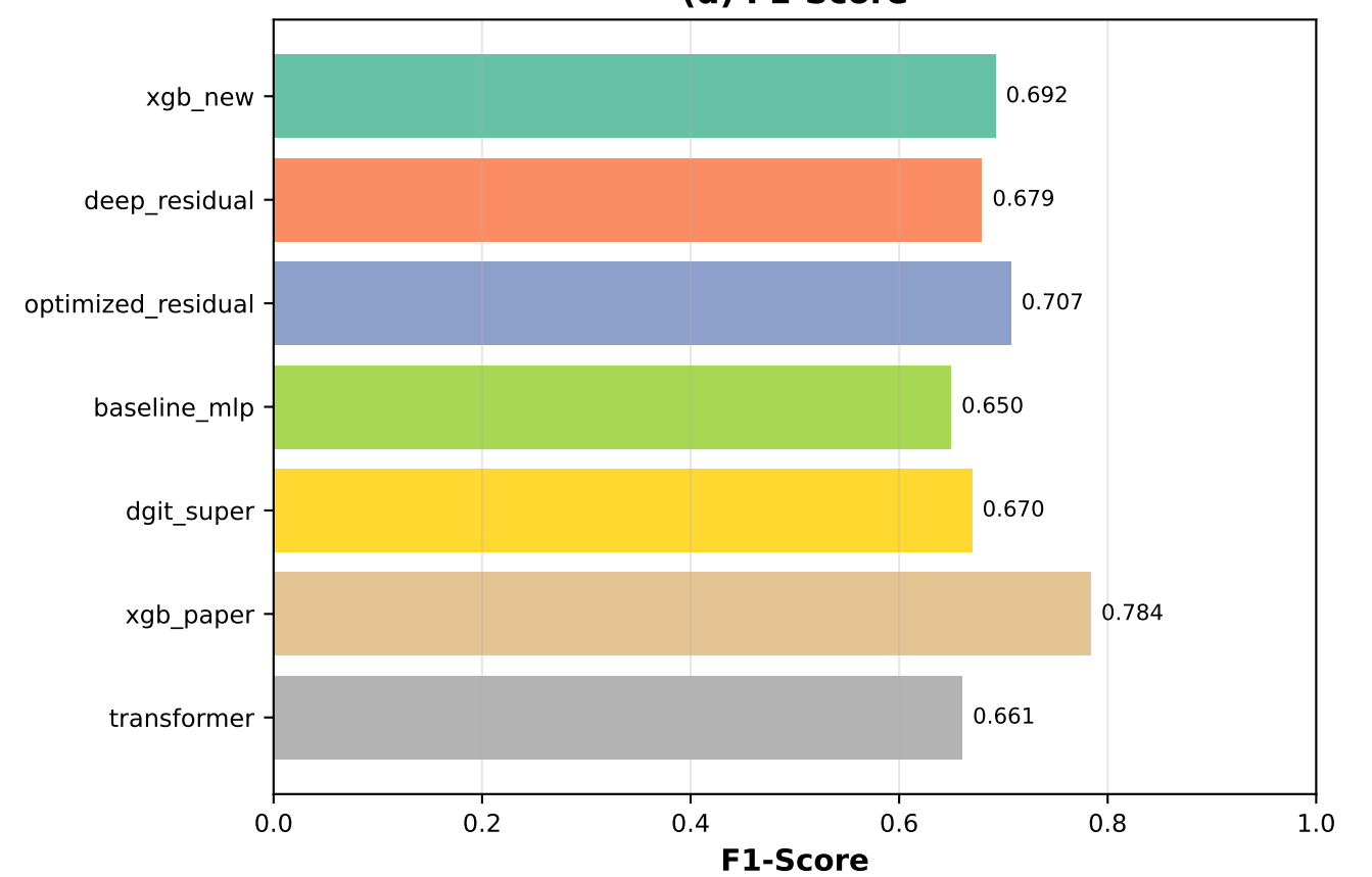
(d) F1-Score
