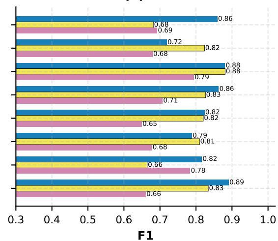
(e) F1
