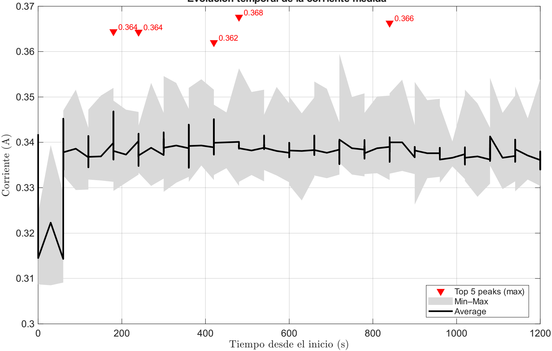
Evolución temporal de la corriente medida
