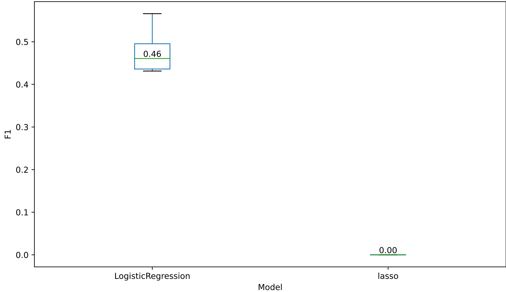
Boxplot for F1
