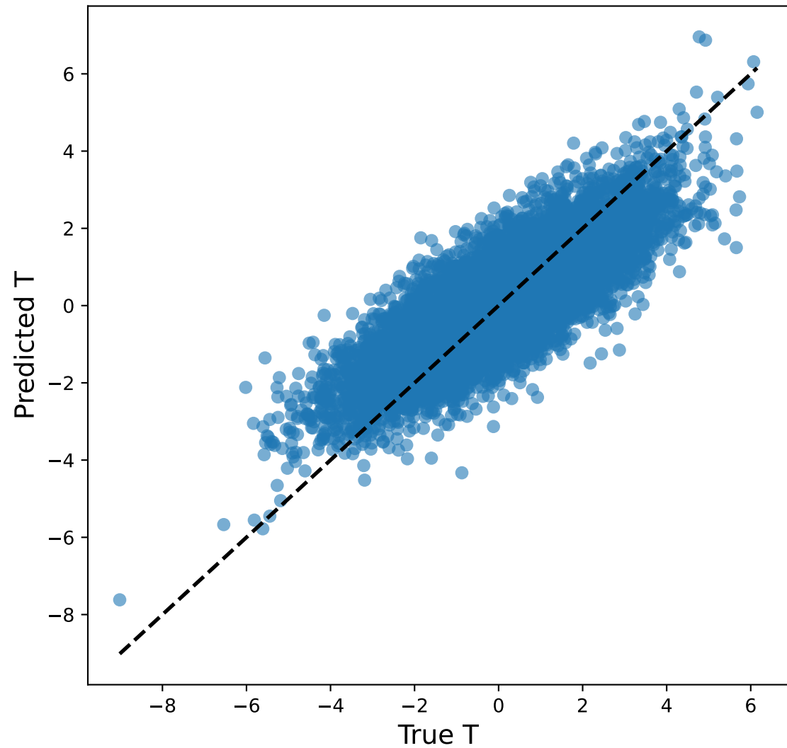
Pure DNN
