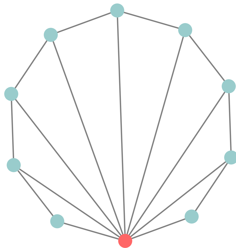
Fan graph
