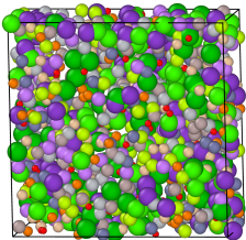
Pure Noise
