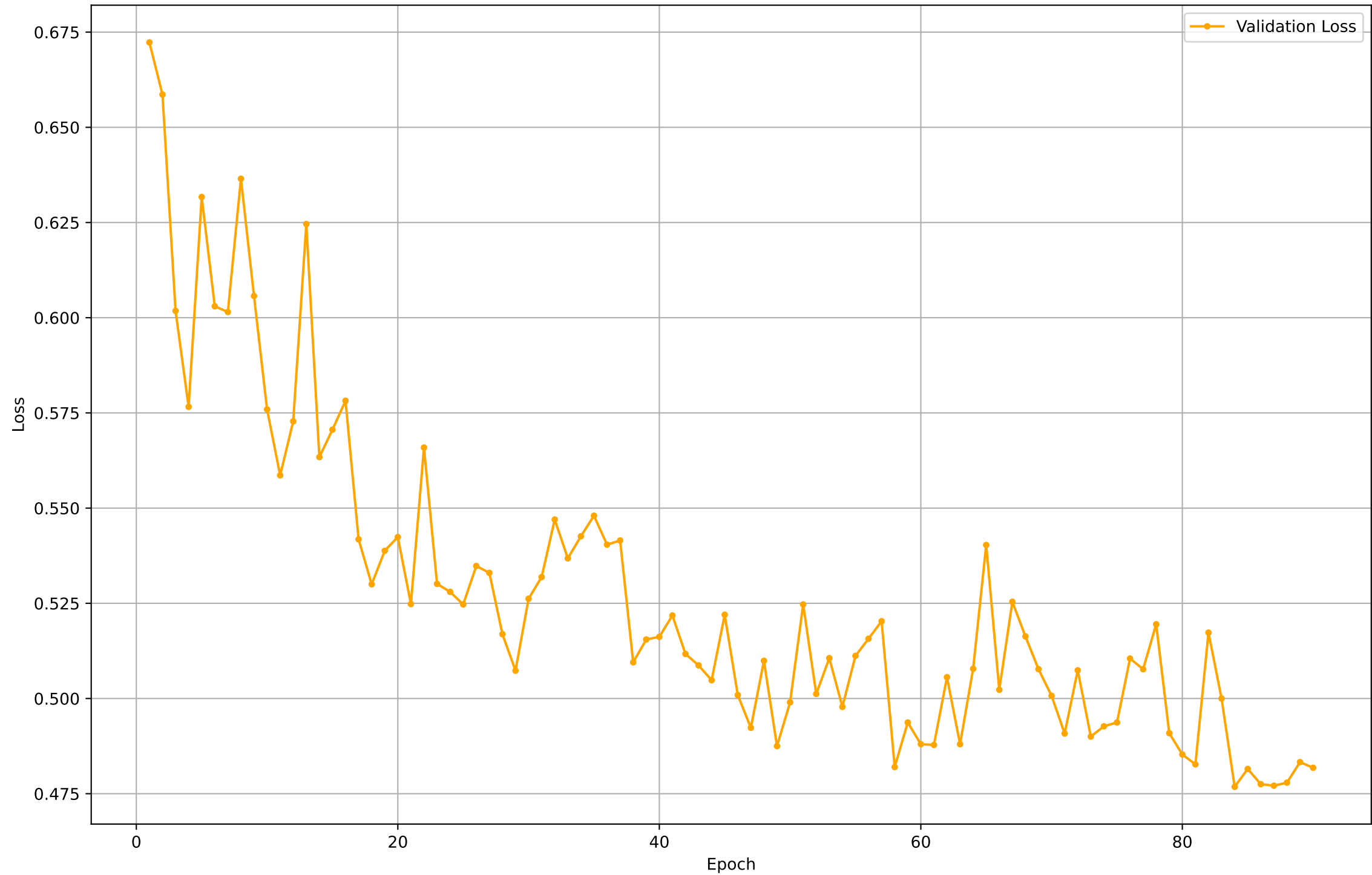
Validation Loss per Epoch
