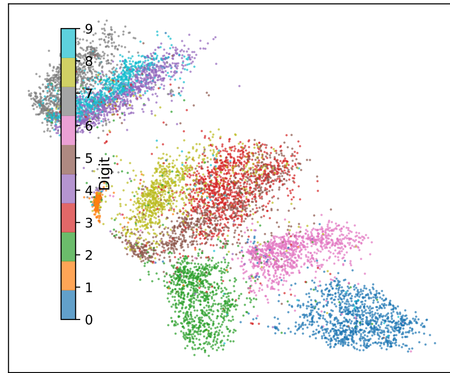
DensMAP \lambda=2.0
