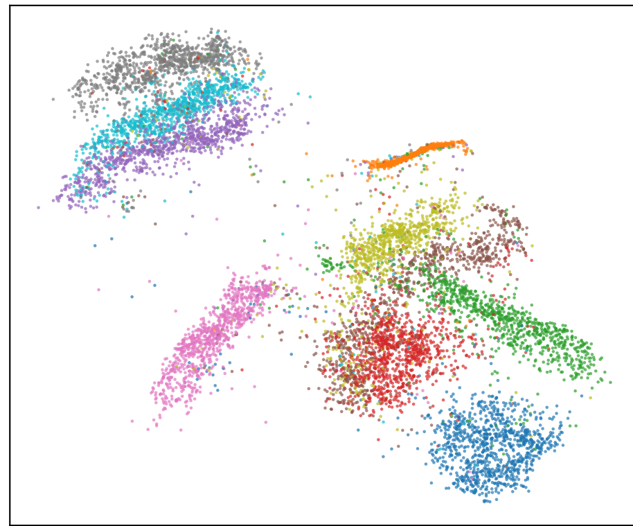
DensMAP \lambda=0.5
