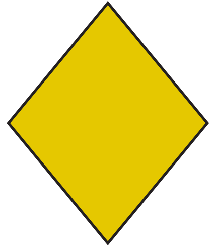
rhombus
