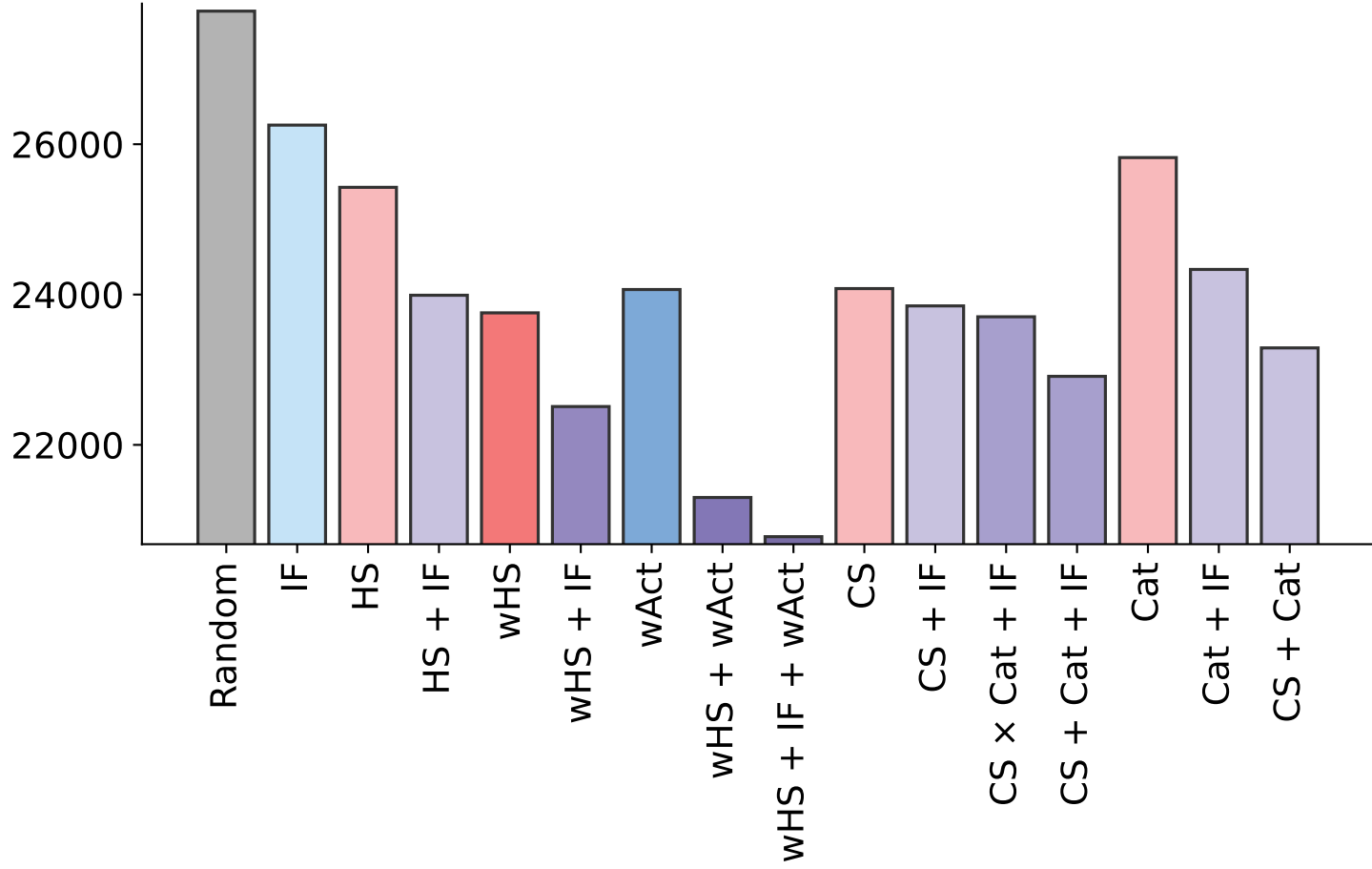
Sum Test NLL (over 5 folds)
